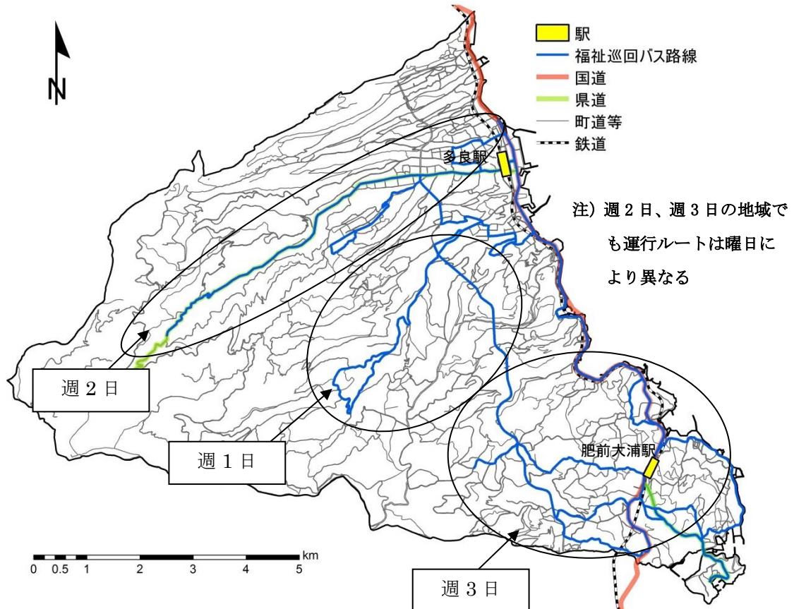
福祉巡回バスの路線網図（平成26年12月現在）
